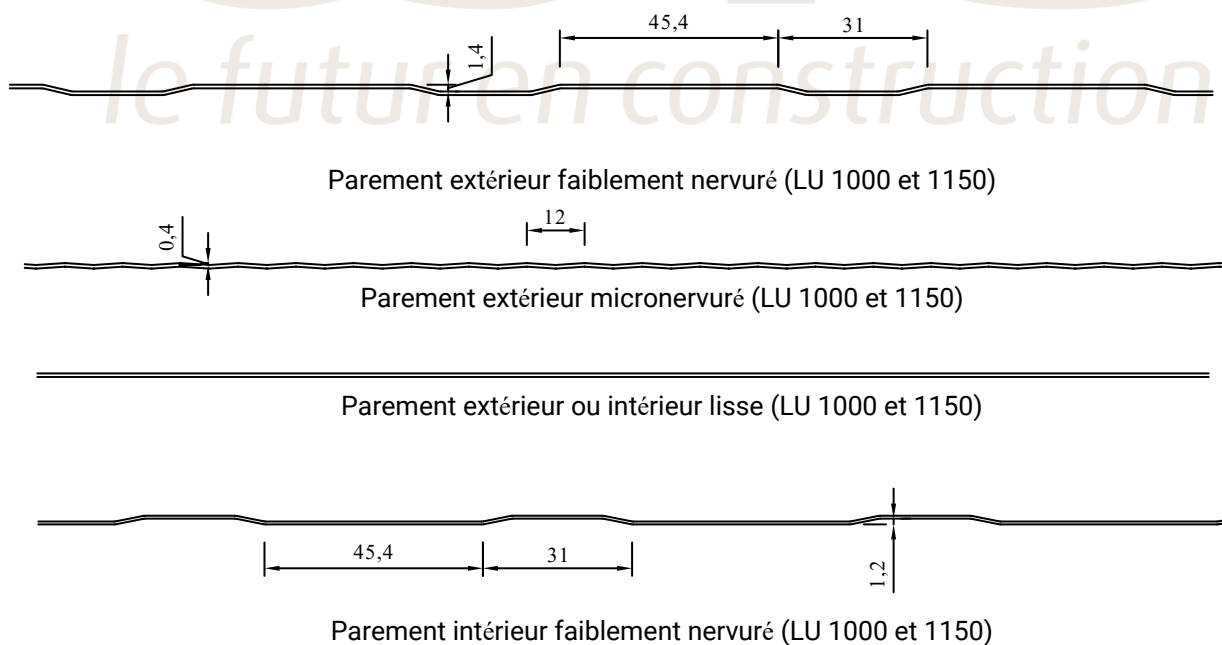
Figure 1 - Panneau Promisol V iQ+ et ses parements (Toutes cotes en mm)
